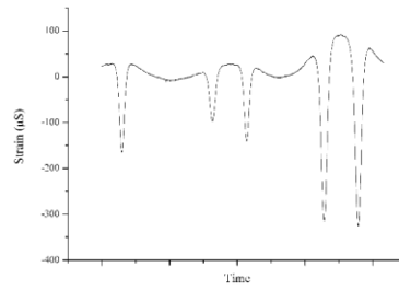
图 9 位置 2 处实测应变时程 Fig. 9 Measured strain on location 2 ( \mu\text{S} )
