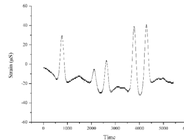
图 12 位置 5 处实测应变时程 Fig. 12 Measured strain on location 5 ( \mu\text{S} )
