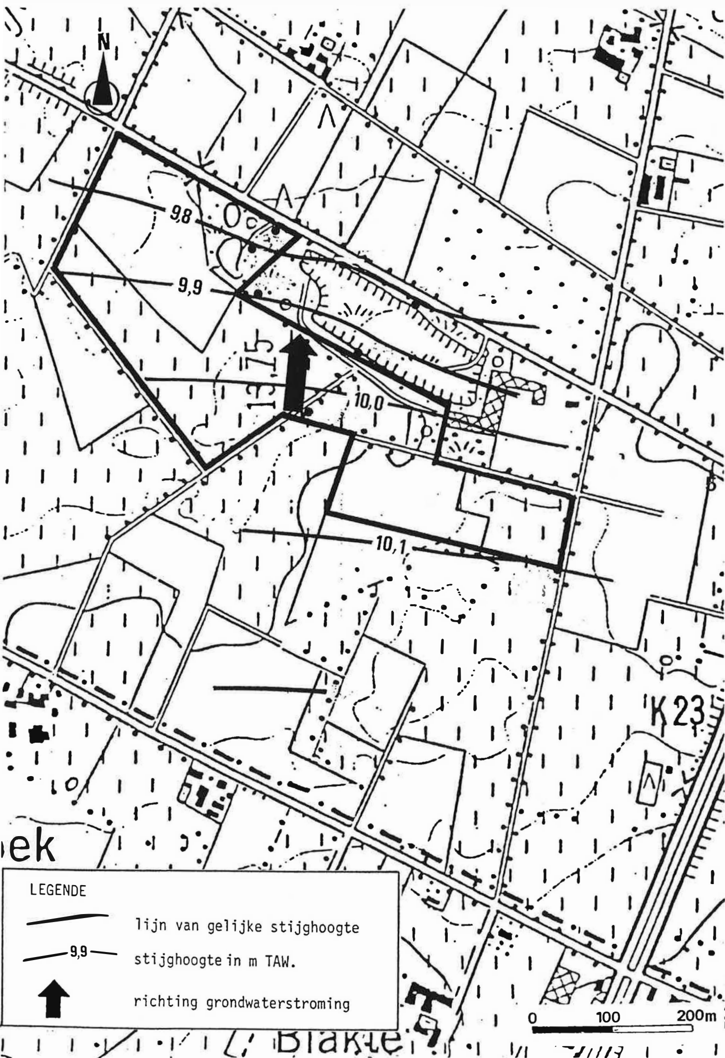
Fig. 11 - Grondwaterstroming in de watervoerende laag onder de Bartoonkley
