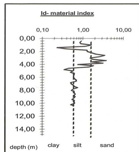
Fig. 1. I_D (DMT1).
