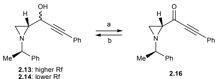
Scheme 7.2: a) Dess-Martin periodinane, CH 2 Cl 2 , 0°C to RT, 4 h (82%); b) L-Selectride, LiBr, THF, -78°C, 1 h ( 2.13 : 52%, 2.14 : 9%, 2.13 + 2.14 : 15%).
