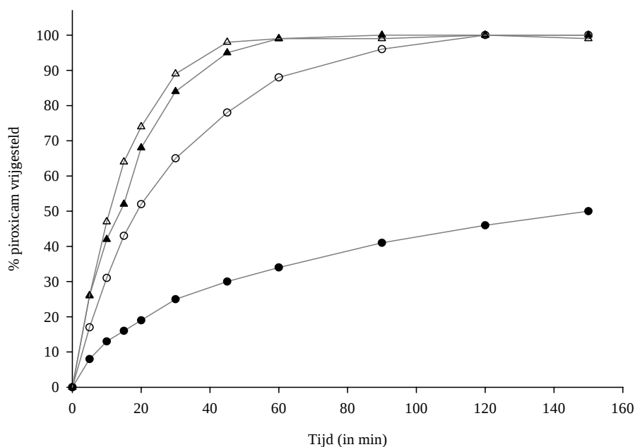
Fig. 2.11: Invloed van het Avicel ® type op de in vitro vrijstelling van piroxicam in fosfaatbuffer pH 6,8. ● Avicel ® PH 101 (referentie); ○ Avicel ® PH 101/CL 611 (1/1), ▲ Avicel ® PH 101/CL 611 (1/3), △ Avicel ® CL 611.
