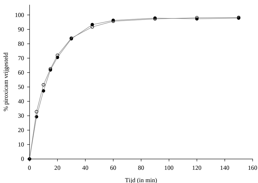
Fig. 2.16: Invloed van de herkomst van piroxicam op de in vitro vrijstelling van piroxicam in fosfaatbuffer pH 6,8. Avicel® PH 101/CL 611 + 2,5 % (g/g) ● Px Sagan; ○ Px Certa.
