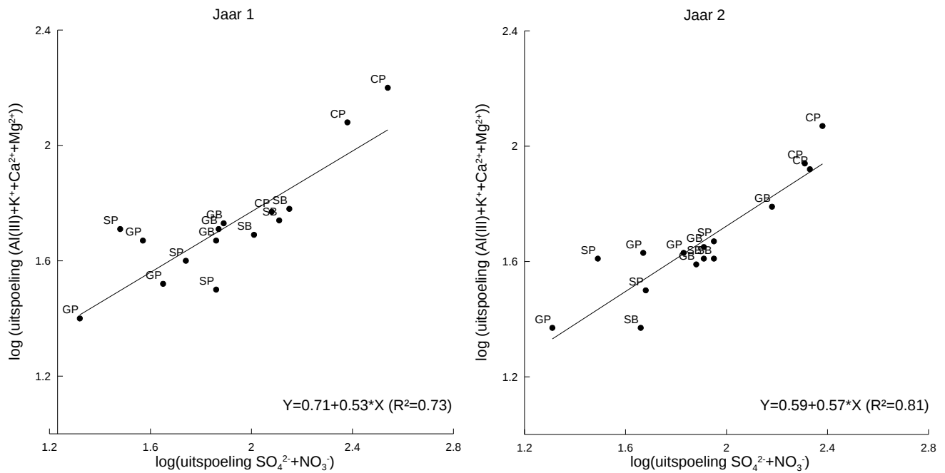
Figuur 14: Relatie tussen de uitspoeling van anionen ( \text{SO}_4^{2-} + \text{NO}_3^- ) en van de kationen ( \text{K}^+ , \text{Ca}^{2+} , \text{Mg}^{2+} , \text{Al(III)} )
